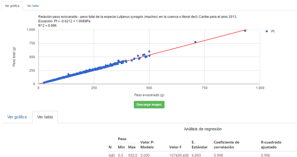
Ilustración 103 Gráfico de regresión lineal con su respectiva tabla de información
