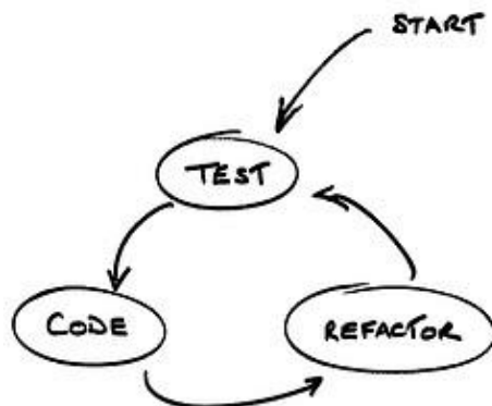
Ilustración 1. Metodología TDD
